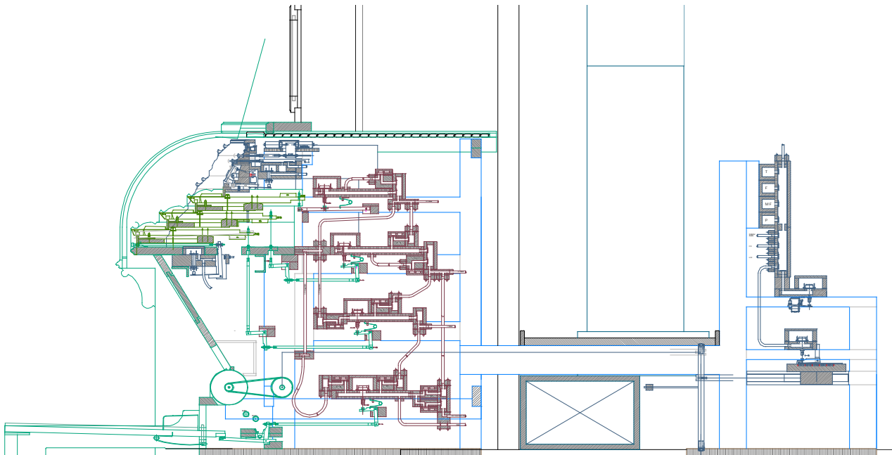
Heidelberg Christuskirche Walcker-Orgel, neuer Spieltisch pneumatisch Seitenschnitt
