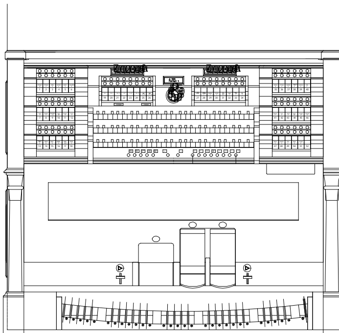
Heidelberg Christuskirche Walcker-Orgel, neuer Spieltisch pneumatisch Seitenschnitt
